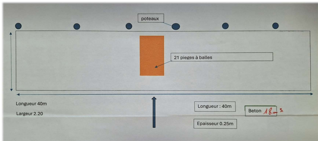
Figure 1 : Plan de la dalle
